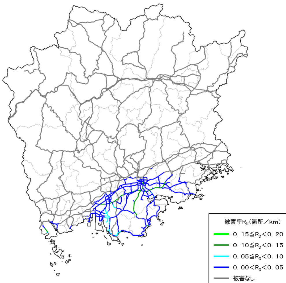
図 5.6.1 道路施設被害
