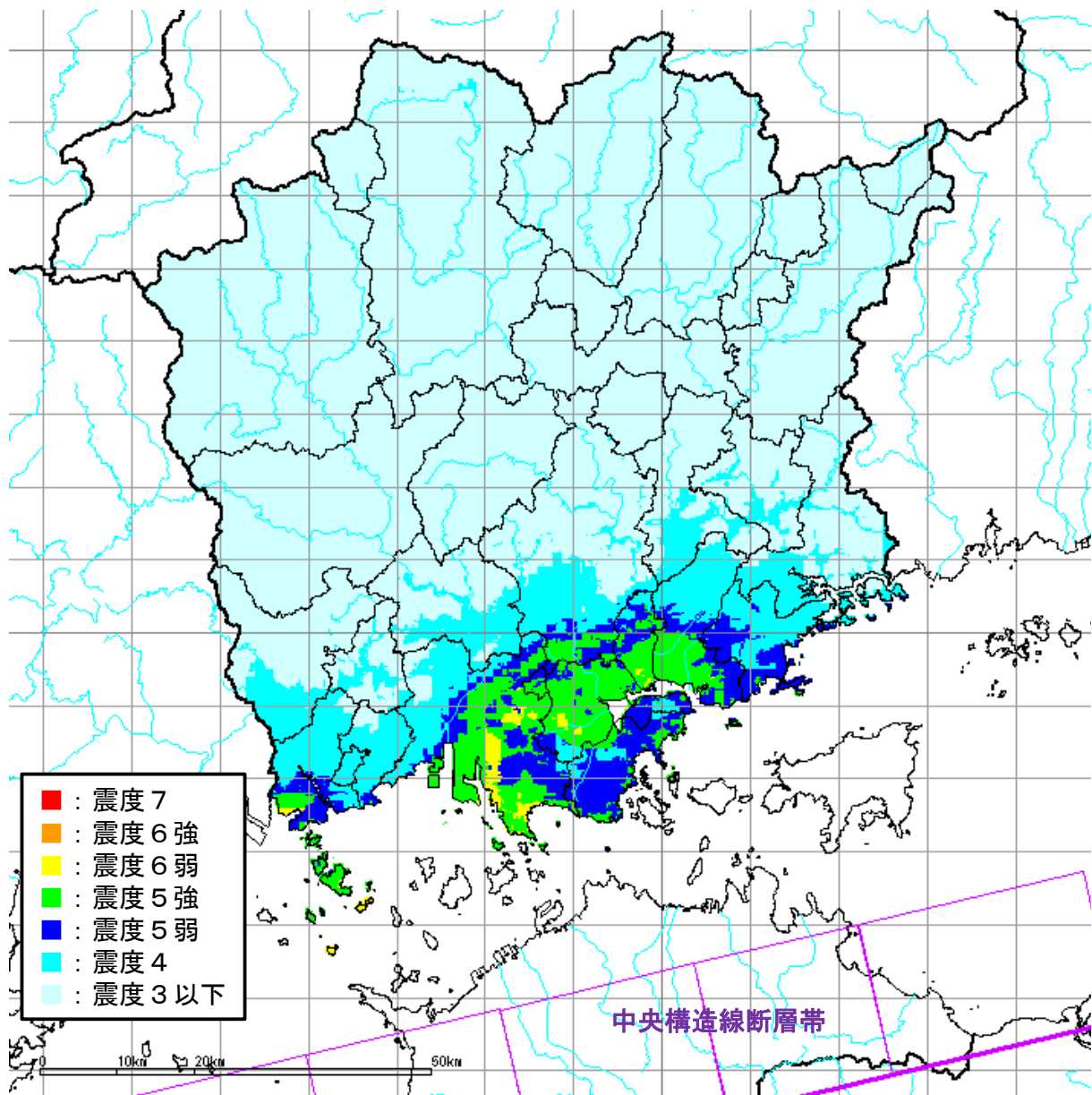
図 5.1.1 震度分布
