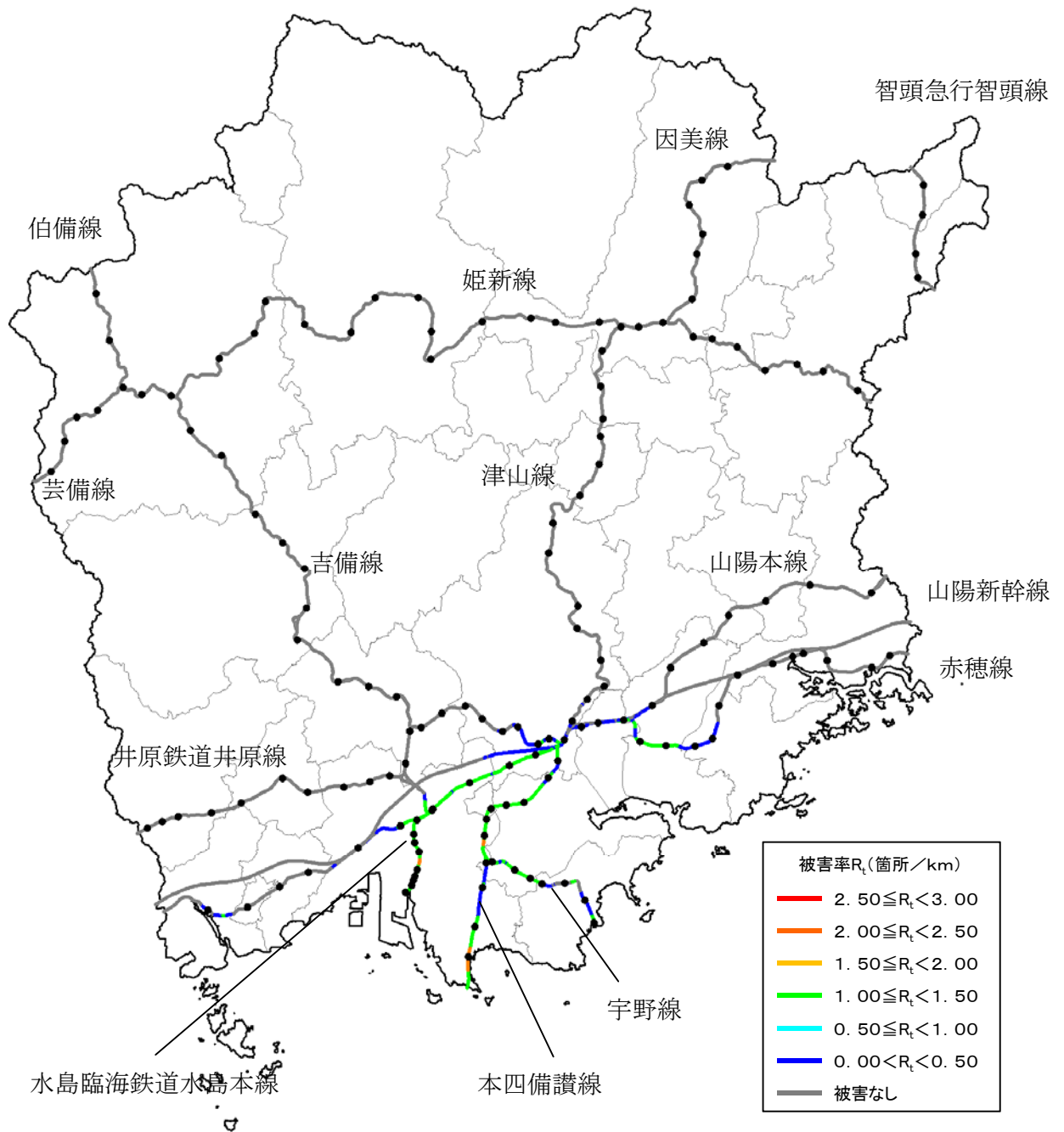
図 5.6.2 鉄道施設被害
