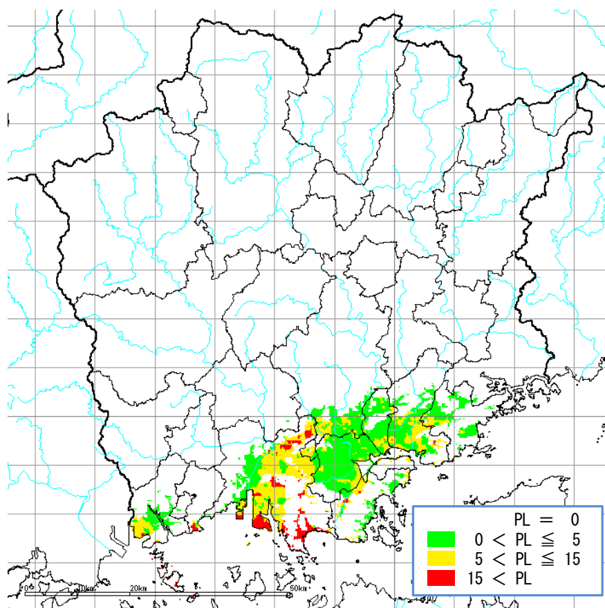
図5.2.1 液状化危険度分布
