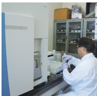
ウランを測定する 高周波誘導結合プラズマ質量分析装置 (ICP-MS)
