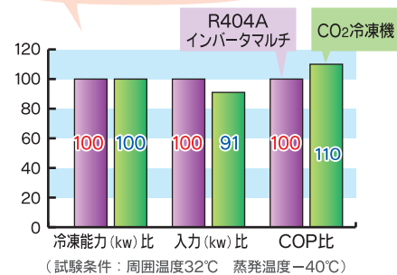
HFC冷媒冷凍機とCO 2 冷媒冷凍機の性能比較図 NEDO「ノンフロン型省エネ冷凍空調システムの開発」事業のデータより環境省作成
