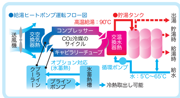
CO 2 冷媒を利用したシステムの一例
