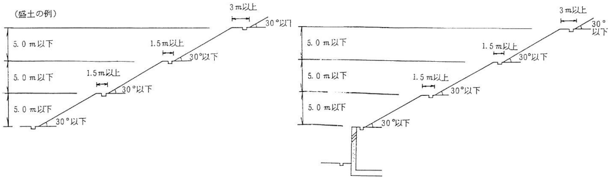
図 盛土の例
