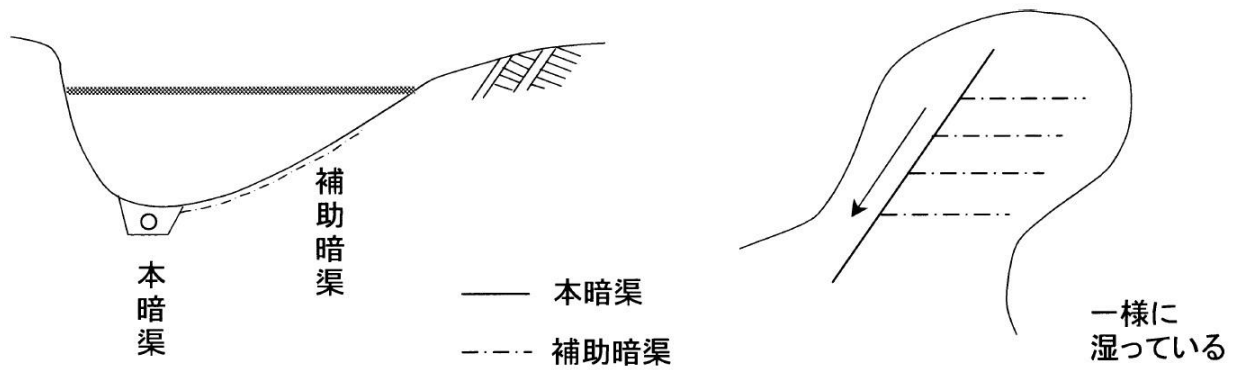
図 くし歯式
