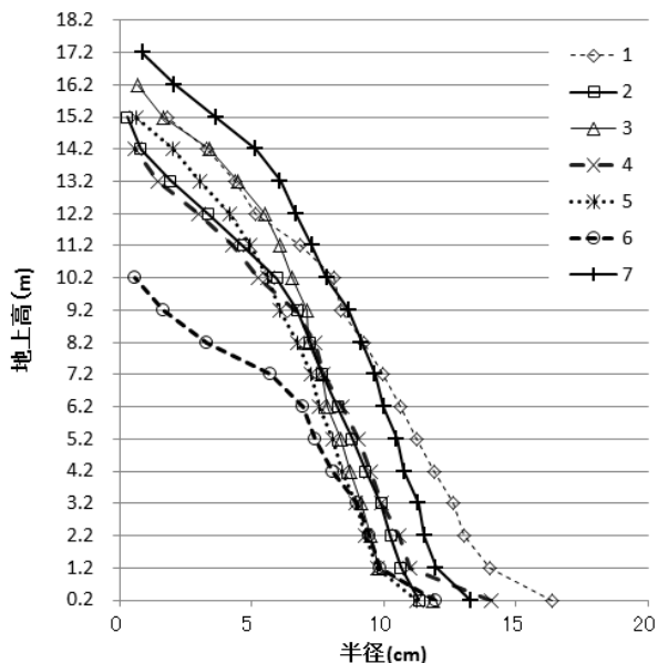
別図三 樹幹曲線 (ヒノキ2-1)
