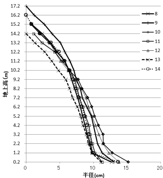
別図四 樹幹曲線 (ヒノキ2-2)
